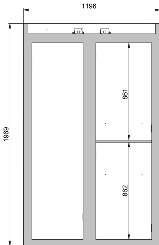
Frontalansicht
