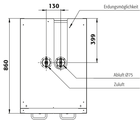
Draufsicht
