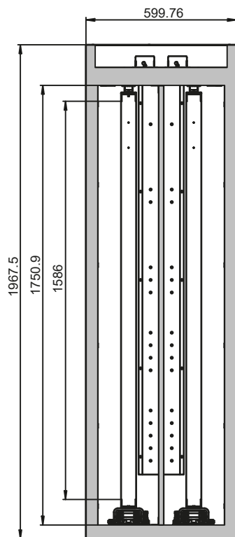
Frontalansicht
