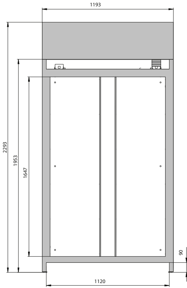
Frontalansicht
